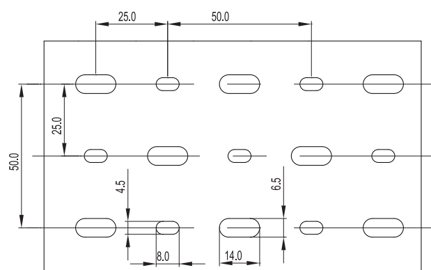
150宽为5排底孔
